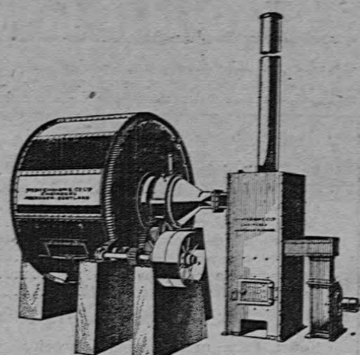
Secadoras de café y cacao. Tipos "Guerdiola", "Okrassa" y "Sterling". Secadoras de cacao con cilindros de aluminio. Diversas capacidades. Todas con cojinetes de bolas.
