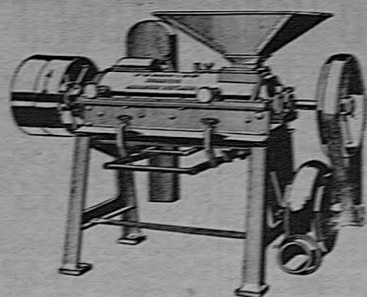
Descascaradora de café con aventador. Último modelo con cojinetes de bolas.
