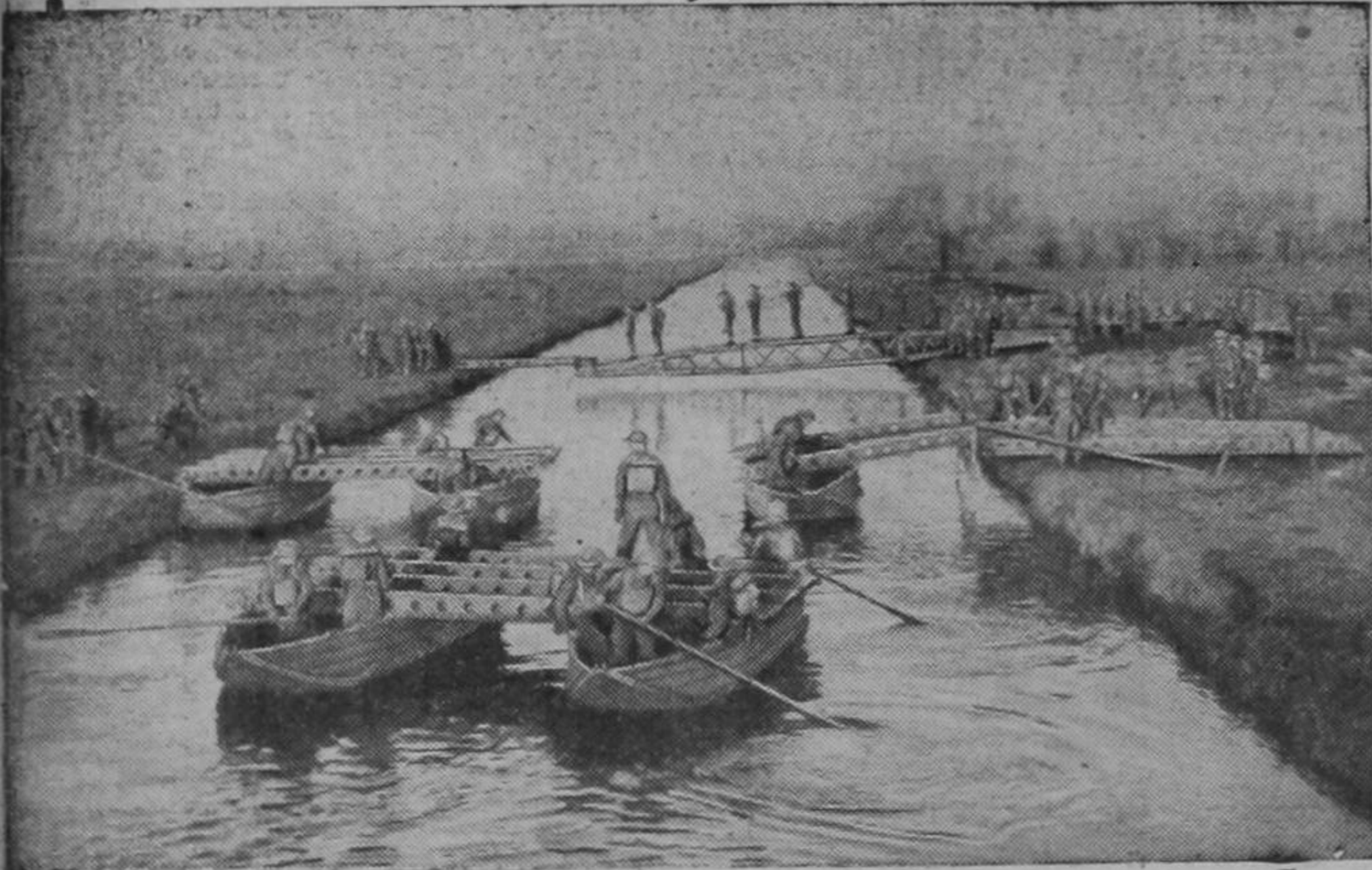
La destrucción de los puentes por un ejército en retirada no presenta ya un obstáculo invencible para uno que avanza. Los Reales Ingenieros Británicos han perfeccionado la rápida construcción de puentes, y esta foto demuestra cómo las secciones de un puente de pontones están siendo colocadas en su posición respectiva.
