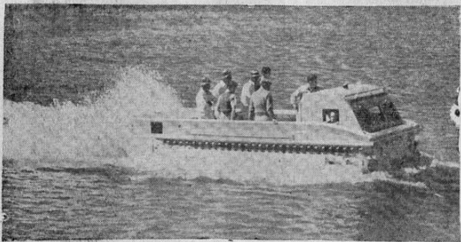
TANQUES AMFIBIOS NORTEAMERICANOS. —Las autoridades navales de los Estados Unidos probaron recientemente este tanque anfibio, cargado con 4,500 libras de bloques de concreto y una tripulación de diez hombres. Mide veinte pies de largo y será de gran utilidad para descargar materiales bélicos de los buques anclados en una bahía.
