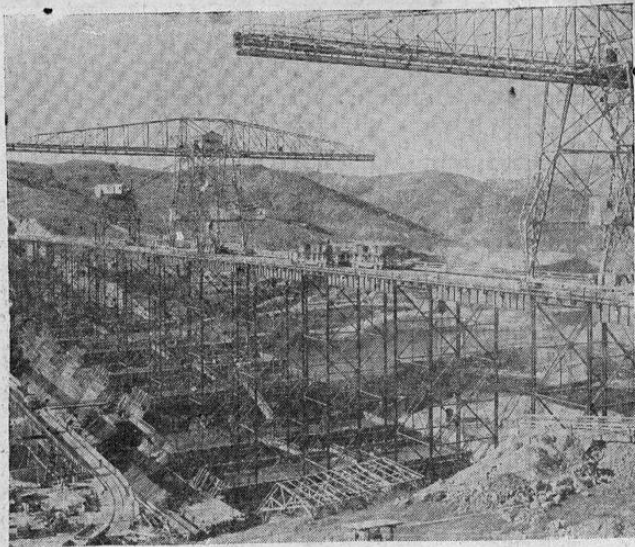
En el Valle Central de California se activan los trabajos de construcción de la nueva Represa Friant sobre el río San Joaquin. Esta obra tiene tan enormes proporciones, que el muro de contención constituye una verdadera montaña de cemento.—(Foto Acme-Editors Press)
