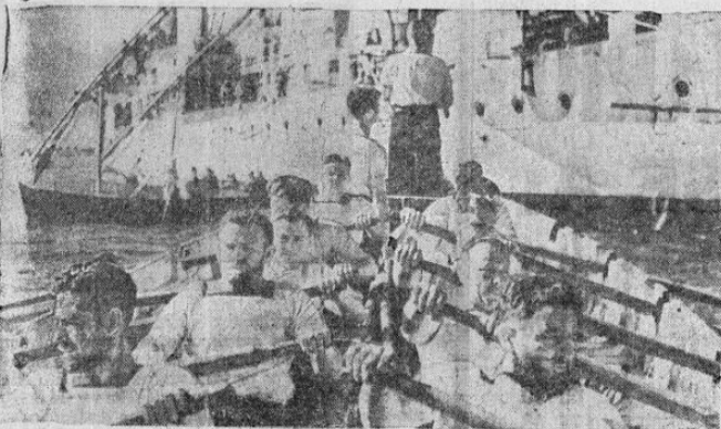
Marineros del "Perth", buque de guerra inglés, regresan a su barco después de haber descansado tras participar en un combate contra buques de guerra italianos en el Mediterráneo. Los ingleses hundieron dos destroyers y tres cruceros de la escuadra de Mussolini.
