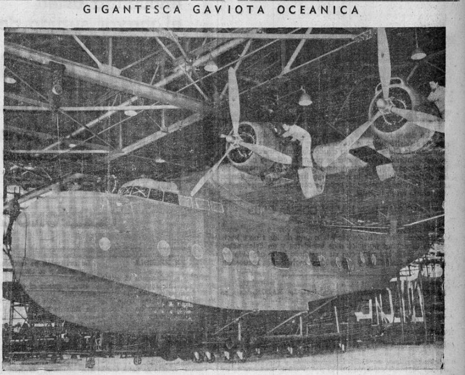
Primero de una serie de gigantescos barcos aéreos de 4 motores que se están construyendo para la "American Export Airlines", destinados al servicio trasatlántico. Este avión de transporte Vought-Sikorsky, fué retratado cuando estaba casi terminado, en una de las fábricas de la "United Aircraft" en Stratford, Connecticut. — (Foto Acme-Editors Press).
