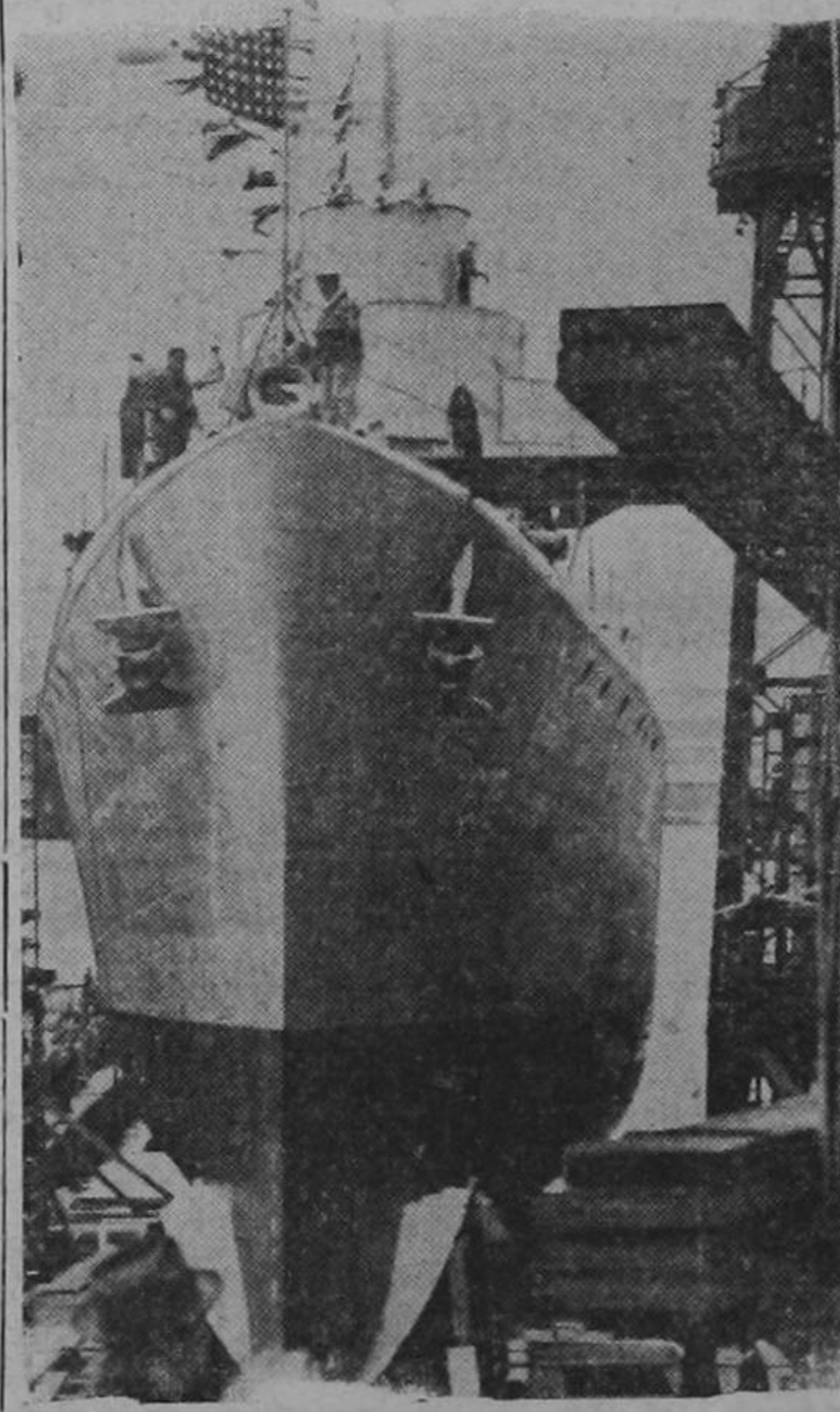
El destroyer norteamericano Herndon, en los momentos de ser botado al agua en Norfolk, Va. exactamente 5 meses y 9 días después de haber sido comenzado. Verdadero record en la construcción de destroyers.
