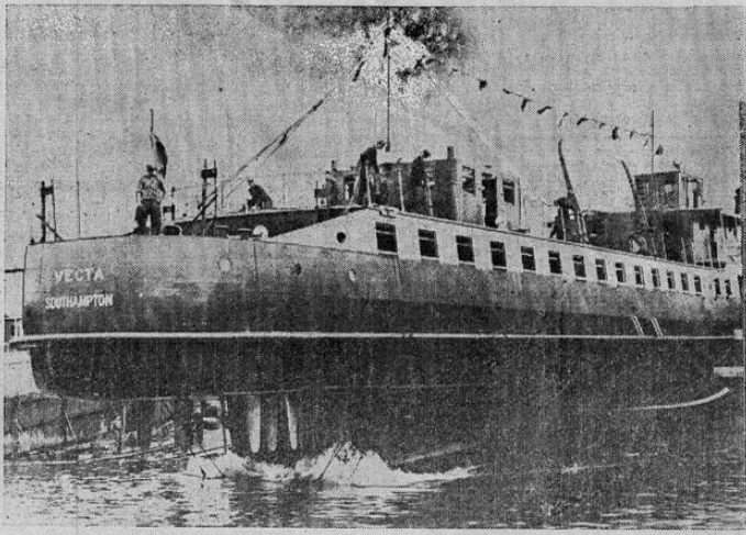
El vapor inglés "Vecta" votado al agua recientemente en Southampton, Inglaterra y que tiene la particularidad de sus hélices verticales, primer buque que lleva esta innovación.
