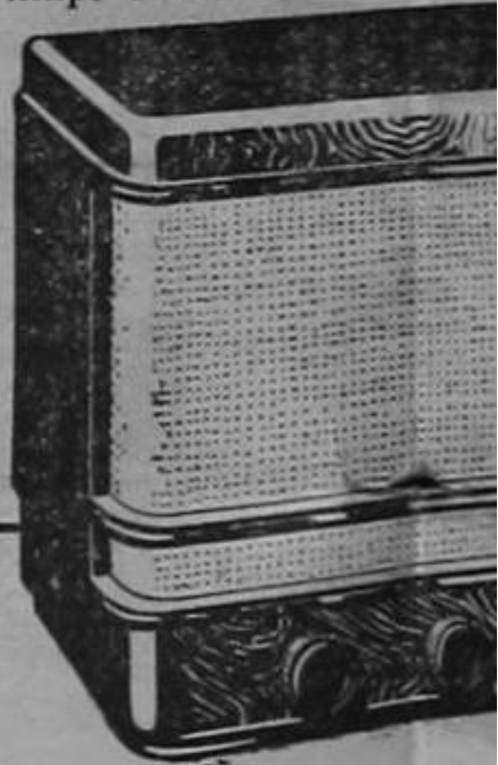
TIPO 313. Superheterodino de 5 v. que asegura una excelente recepción en onda corta, gracias al Silentodo en el paso de R. F. y al nuevo tubo triodo-hexodo como estabilizador de frecuencia. Otras características: compensador de sintonización de Punto Luminoso y gama de ondas ininterrumpida de 13.5 — 570 m.
