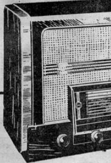
TIPO 316. Superheterodino de banda spread de B.V. con selector automático de banda, sintonizador de banda spread de permeabilidad, dial calibrado para el bandspread en las bandas de 13, 16, 20, 25 y 30 m. Alta sensibilidad y bajo nivel de ruidos, gracias al tubo Silenado y al tubo triodo basado para la estabilización de la frecuencia. Gama de onda 13,6 - 585 m.
