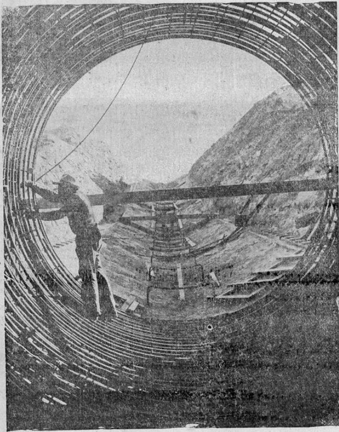
Estas son las costillas de acero preparadas para reforzar el hormigón colocado en el enorme sifón de 12 pies de diámetro que se construye en el Canal de Madera. Tres de estos conductos constituirán un canal que unirá dos tintos zonas en el Valle Central, en Friant, California
