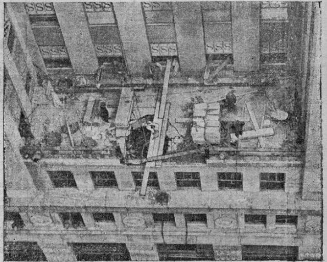
Varios trabajadores escaparon milagrosamente con vida cuando un bloque de terra-cotta que pesaba media tonelada, se cayó desde el piso veintinueve al romperse el cable que lo llevaba al piso sesentiocho del edificio más alto del mundo, el del Banco de Manhattan, que está a punto de terminarse en Wall Street. El enorme pedrusco atravesó tres pisos e hizo este enorme hueco en el noveno piso. Tres personas resultaron fuertemente heridas.
