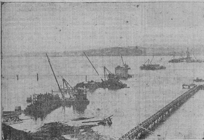
En la foto se ve el estado actual del nuevo puente del ferrocarril Sur-Pacífico que une las dos orillas de la bahía de San Francisco, desde Suisun Point hasta Army Point. Tendrá una longitud de 5.598 pies y costará doce millones de dólares
