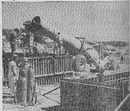
Un tipo nuevo de mezcladora de cemento está ayudando a apresurar la construcción en un proyecto de construcción de viviendas en masa, en St. Louis, Estado de Misuri. Girando de derecha a izquierda el barril, de 24 pies de largo mezcla arena, cemento y grava a medida que avanza por su propio motor al sitio de construcción. Mezcla siete yardas cúbicas a la vez, y así los contratistas pueden usar más del triple que la cantidad producida por las mezcladoras corrientes. Si se necesita, puede elevar su barril a una altura de 23 pies para descargar su contenido. La mezcladora, que se maneja mediante botones mecánicos, pesa 32.400 libras.
