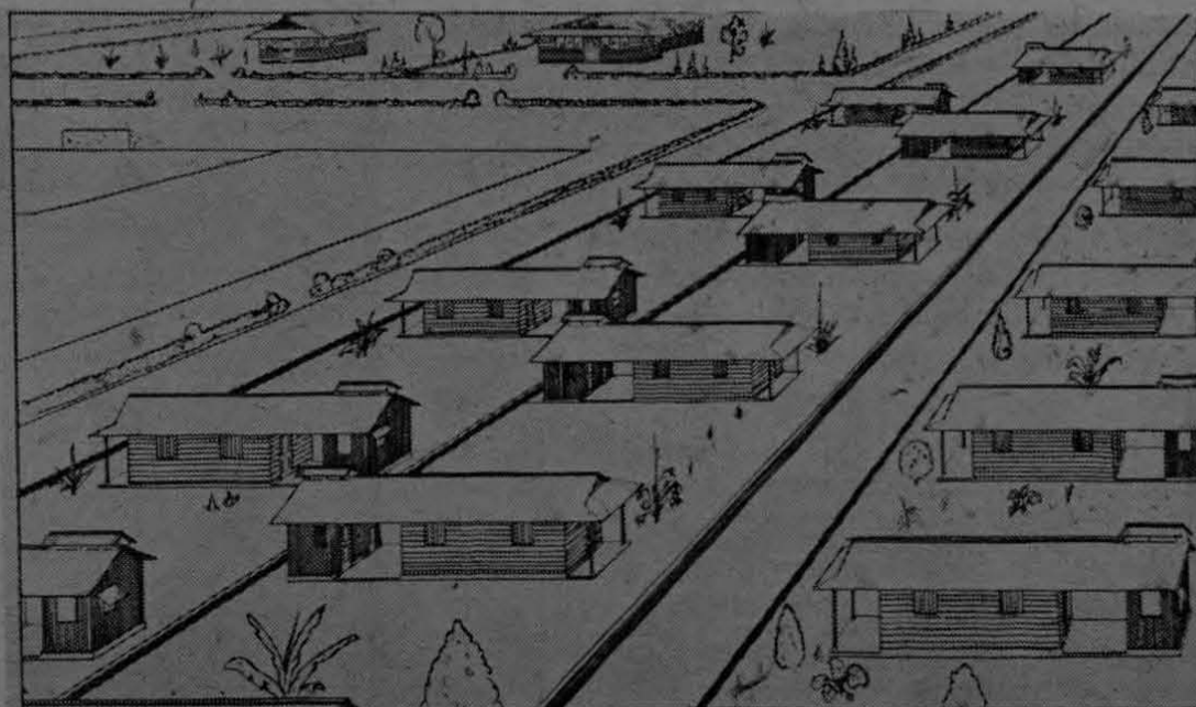
PERSPECTIVA MOSTRANDO UNA SECCION DEL AREA PARA VIVIENDAS DE TRABAJADORES (EDIFICIOS UNIFAMILIARES) SEGUN PROYECTO PARA FUTURAS FINCAS Escala 1:250 Dibujo No. 14-55
