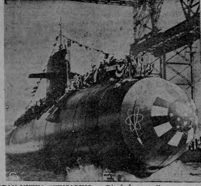
BOTAN NUEVO SUBMARINO. — Diseñado para disparar proyec- tiles balísticos Polaris, el submarino nuclear "Theodore Roose- velt", de 880 pies, es botado en Mare Island, Vallejo, California. Este submarino, que es el primero de su clase en ser construido en la Costa Occidental, está equipado con 16 tubos disparadores para acomodar los proyectiles
