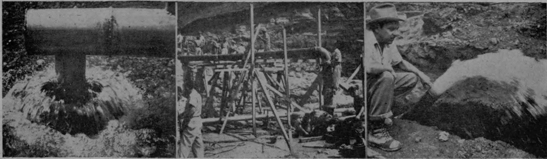
Las gráficas de Artavia nos muestran: 1º La perforación N° 2 "El Papá". Se observará un tubo vertical dentro de la perforación, unido a otro que lleva el agua al tubo de hierro de la cañería. — N° 2 Armazón de madera para sostener la tubería que lleva el agua al tubo de hierro. Se aprecia parte de la bomba y del motor. — N° 3 Perforación N° 6, en plena producción. Un potente chorro de agua es lanzado. Se conectará oportunamente a la cañería.
