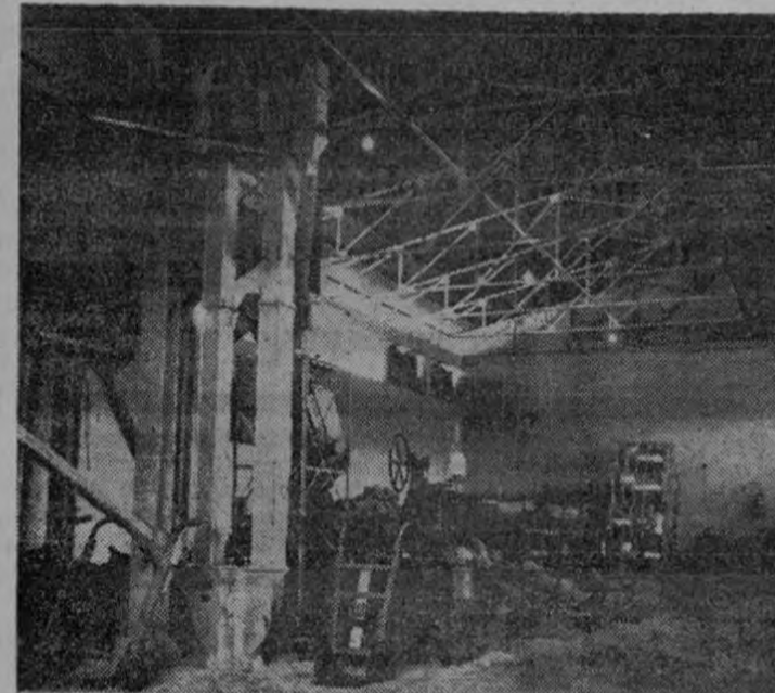
Vista parcial del interior, en la cual se aprecia la maquinaria para ensacar y pesar el grano. La secadora fue construida en 1957 a un costo aproximado de un millón de colones. Parte de la maquinaria fue diseñada por funcionarios del Consejo y fabricada en los talleres de la Institución.
