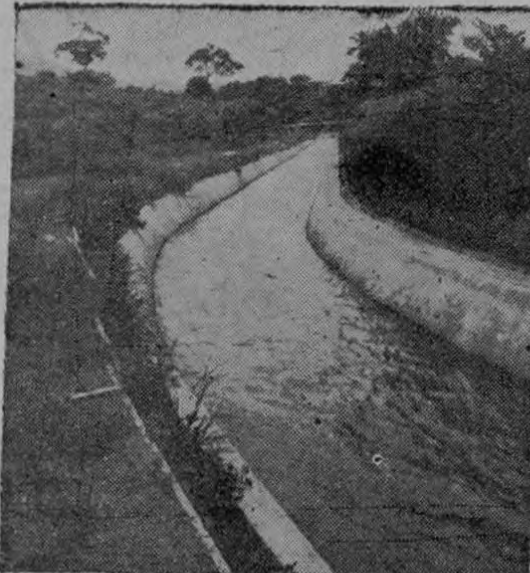
Radas por donde transcurrir el agua cuando la topografía lo permite.
