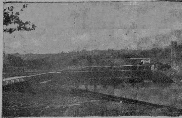
Estructura de entrada a la tubería forzada, prevista de rejillas y otros dispositivos de limpieza.
