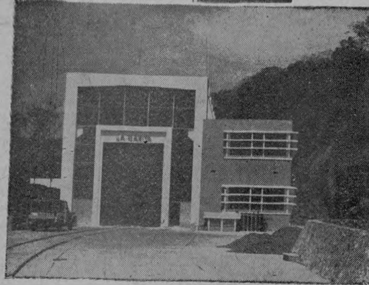
Una de las obras más hermosas de La Garita. La excavación realizada fue uno de los puntos más difíciles del Proyecto. Está hecha para incluir la tubería de la ampliación a 60.000 KW.
