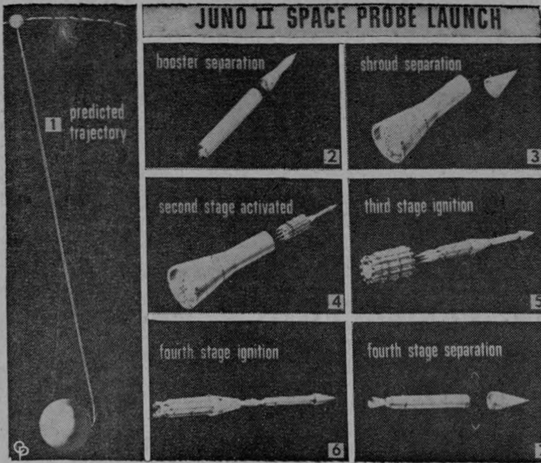
Estos dibujos del ejército de Estados Unidos ilustran la trayectoria pronosticada (1) y la separación del proyectil Juno Segundo que disparó el satelóide Pionero IV hacia el espacio. El satélite se espera que pase a unas 35.000 millas de separación de la luna, y siga su curso hasta convertirse en satélite del sol. El cohete fue disparado en Cabo Cañaveral.
