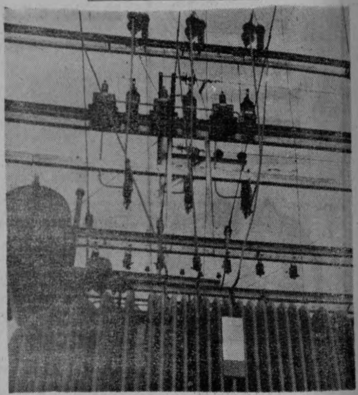
Una vista parcial del transformador de 1.500 KW instalado en la ciudad de Grecia, y que proporciona inmejorable corriente eléctrica a la población
