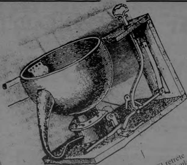
Retrete de válvula sin caja
