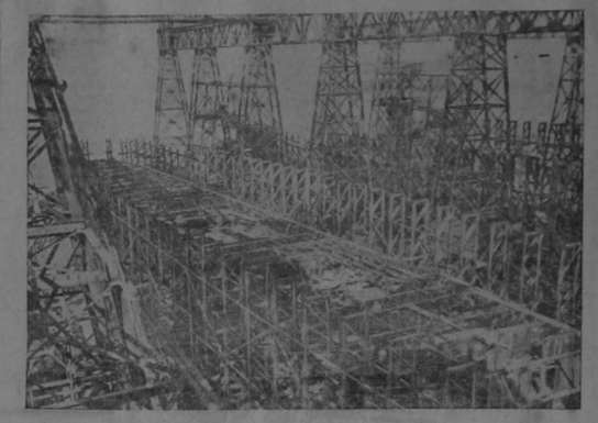
"El U.S.S. Pensacola", el nuevo crucero de 16000 toneladas de desplazamiento q' la Armada norteamericana está a punto de terminar en los astilleros de Brooklyn, N. Y. Este es el primero de los grandes cruceros que está construyendo el gobierno norteamericano después de la conferencia del desarme.
