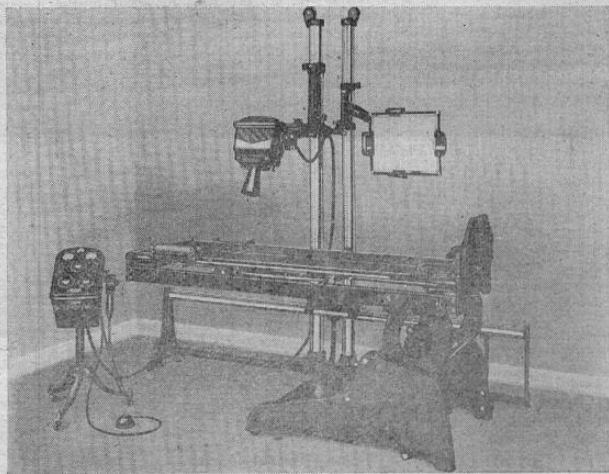
Aparato pequeño. Capacidad 80 K.V. — 80 Ma.
