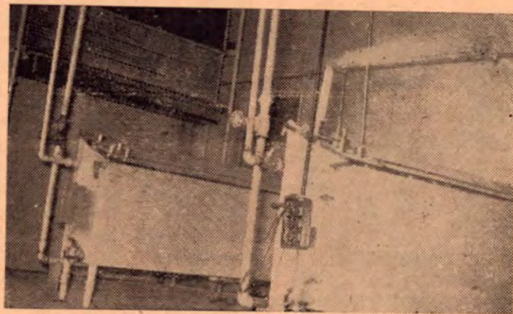
Sala de Pasteurización y Enfriadora de la Leche Pasteurizada
