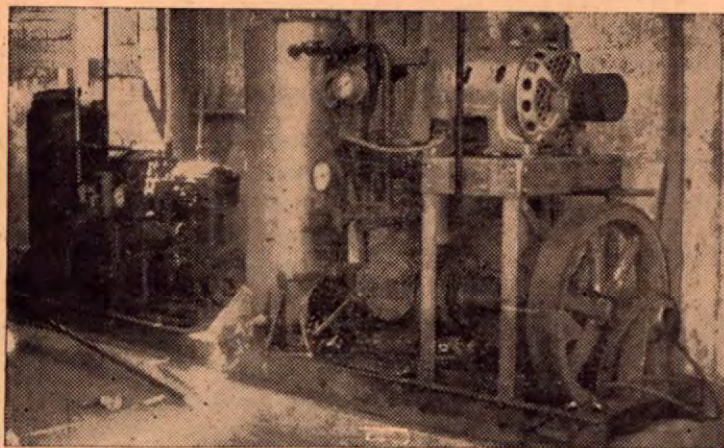
COMPRESORES DE REFRIGERACION (Sala de máquinas)
