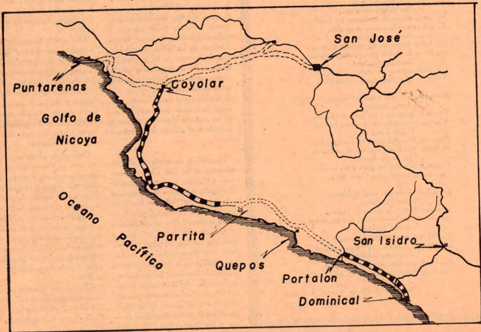
— Esquema gráfico del proyecto del Ferrocarril Quepos - Orotina —
