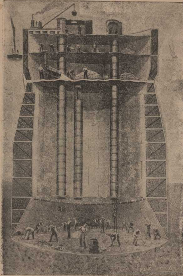
Este cajón flotante, que tomamos como ejemplo de los trabajos que supone la construcción de un puente, sirvió para echar los cimientos a las dos columnas del célebre puente de Forth. El grabado muestra como pueden trabajar los obreros en el interior del cajón y cómo tienen abundante aire respirable por los tubos que desde la superficie llegan al fondo. Por dentro de uno de ellos va una escalera. Otro tubo sirve para subir el material extraído e inútil a la construcción. Si el lecho del río es cenagoso el légamo se extrae mediante aire comprimido y este mismo agente mantiene segura la cámara contra la presión del agua, la cual, si no fuese por esto llegaría a romper el cajón.
